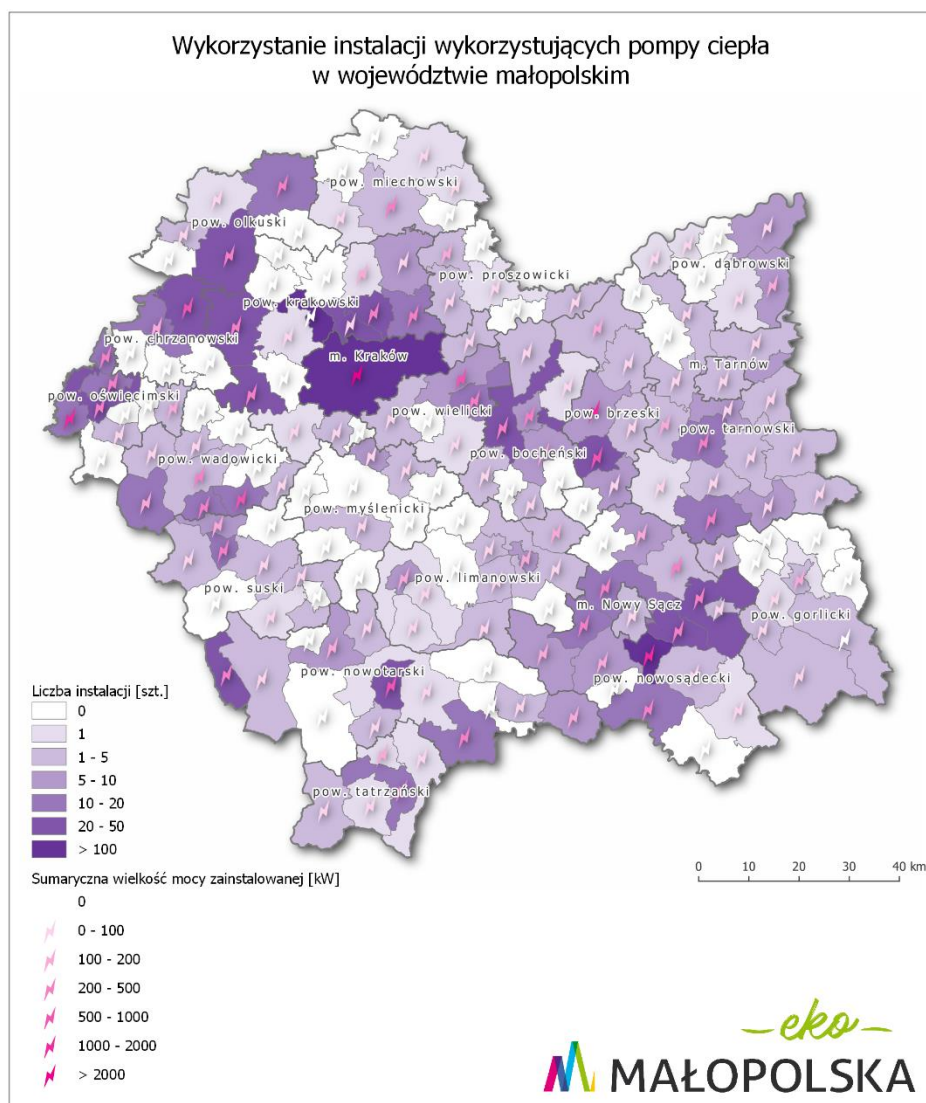
Rysunek 67. Instalacje wykorzystujące pompy ciepła w województwie małopolskim (opracowanie własne)
